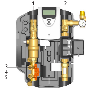
Beispiel: Solarstation mit Spül- und Befüllinheit
