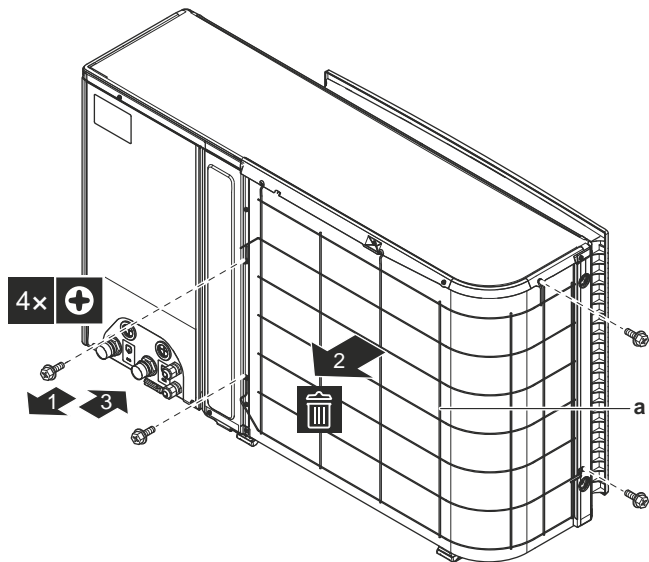
a Ansaugluftgitter
