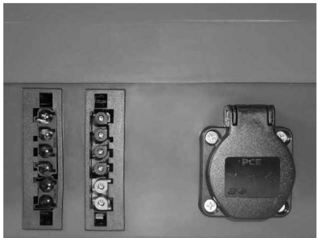
Abb. 12 - Brenner / zwei 6 Pin-konnectore,- links Spannung, rechts Fühler und Steckdose für Förderschnecke
