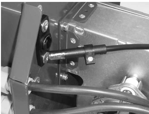
Abb. 6 - Photozelle - Vorsicht auf richtige Ori- entierung – es wird empfohlen, die Zelle mindes- tens einmal jährlich zu reinigen
