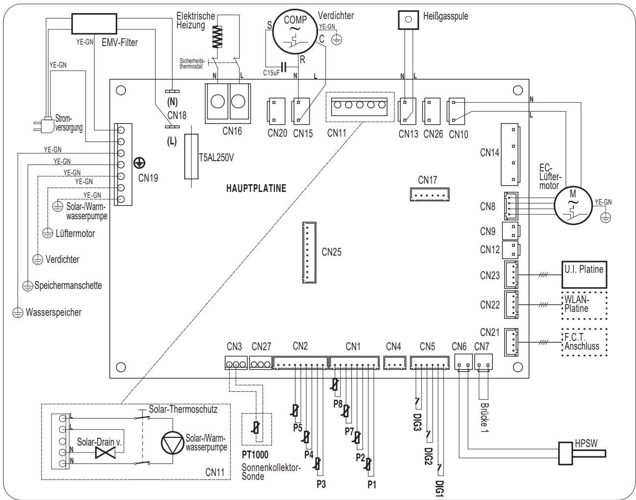
Abb. 26- Beispiellektroschaltplan
