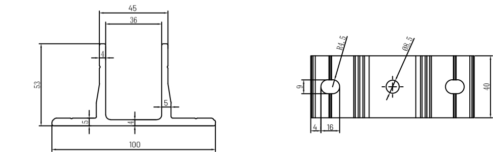
Stütze
