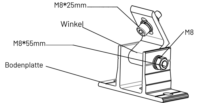
Winkel
