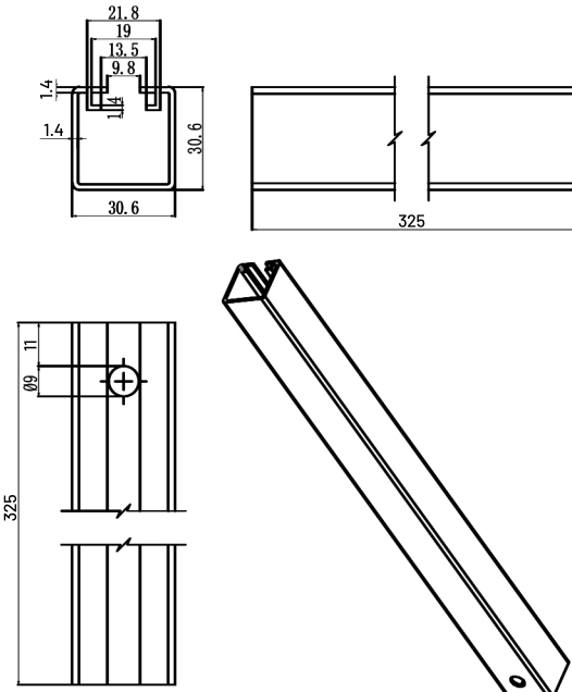
Innenstütze
